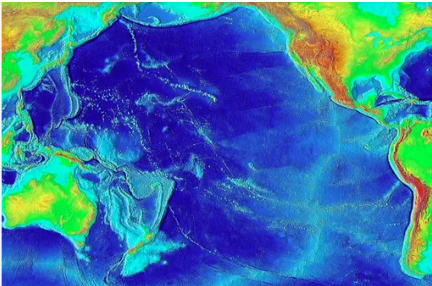
Карта рельефа дна Тихого океана. Области океанических впадин выделены темно-синим цветом ozeraireki.ru
